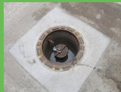
Spill bucket
